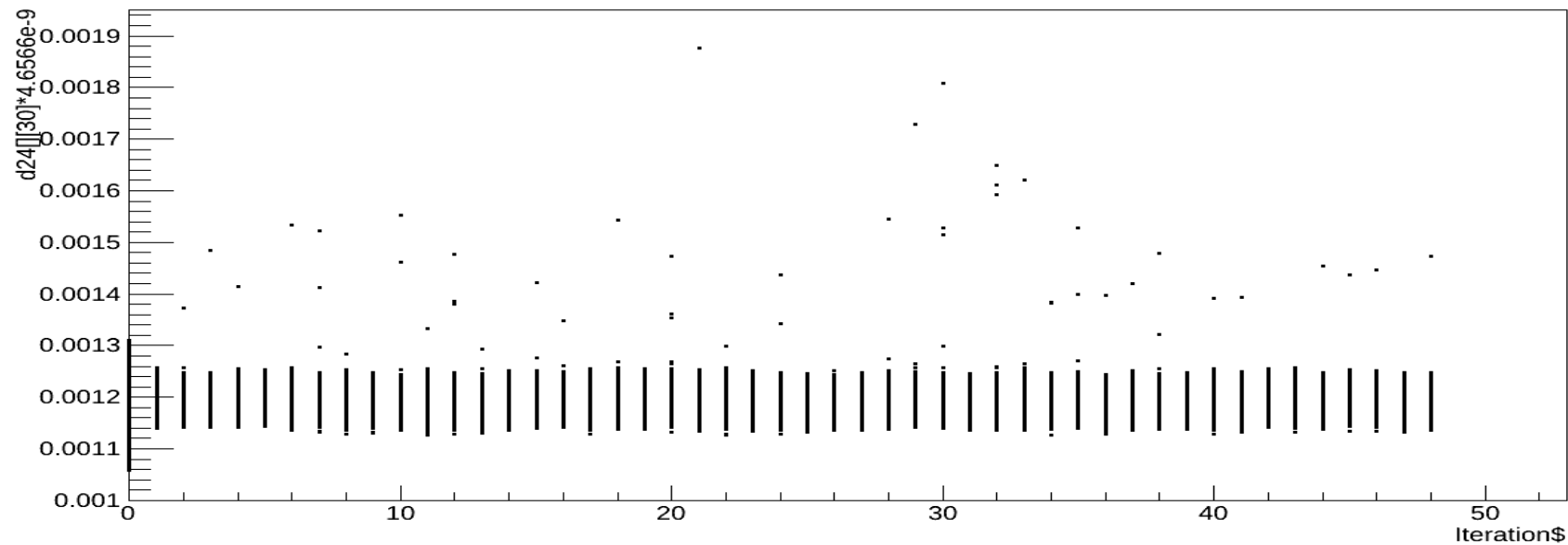
d24[[30]*4.6566e-9:Iteration$
